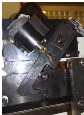
Blocco Lama elettromagnetico di sicurezza
